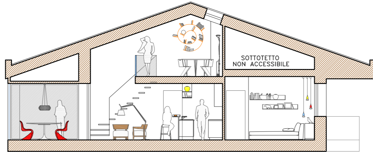
SEZIONE A-A
