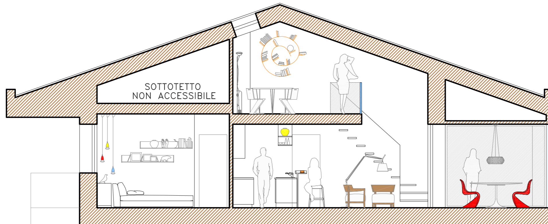
SEZIONE A-A
