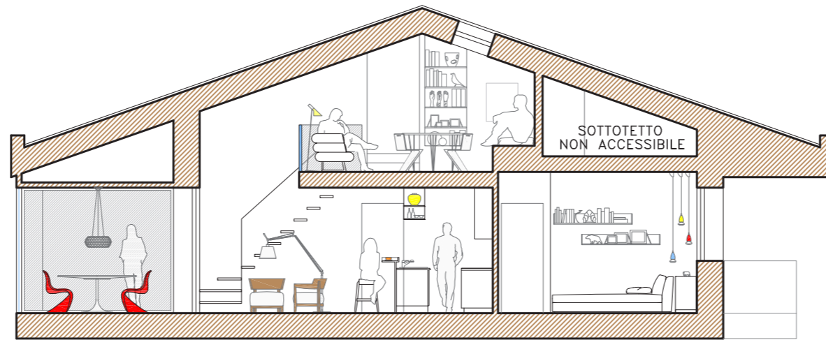
SEZIONE A-A
