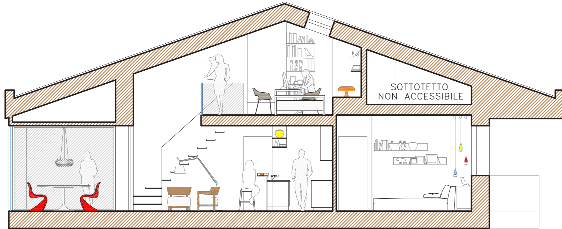
SEZIONE A-A
